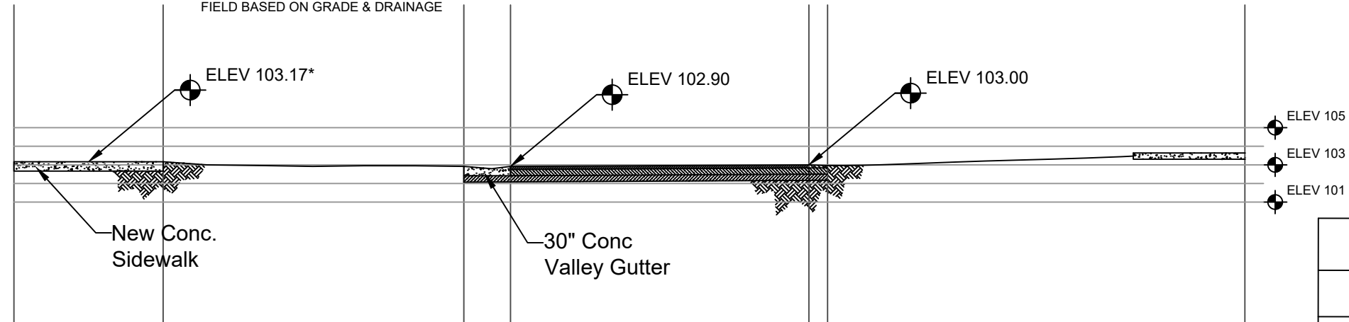
CROSS SECTION STA 02+50
