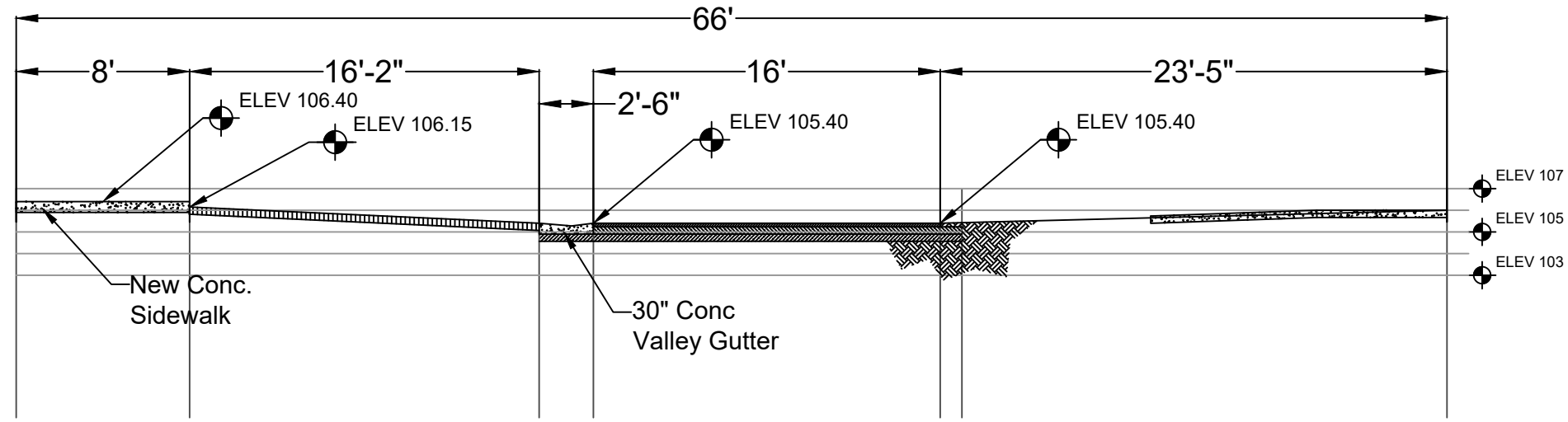
CROSS SECTION STA 01+50
