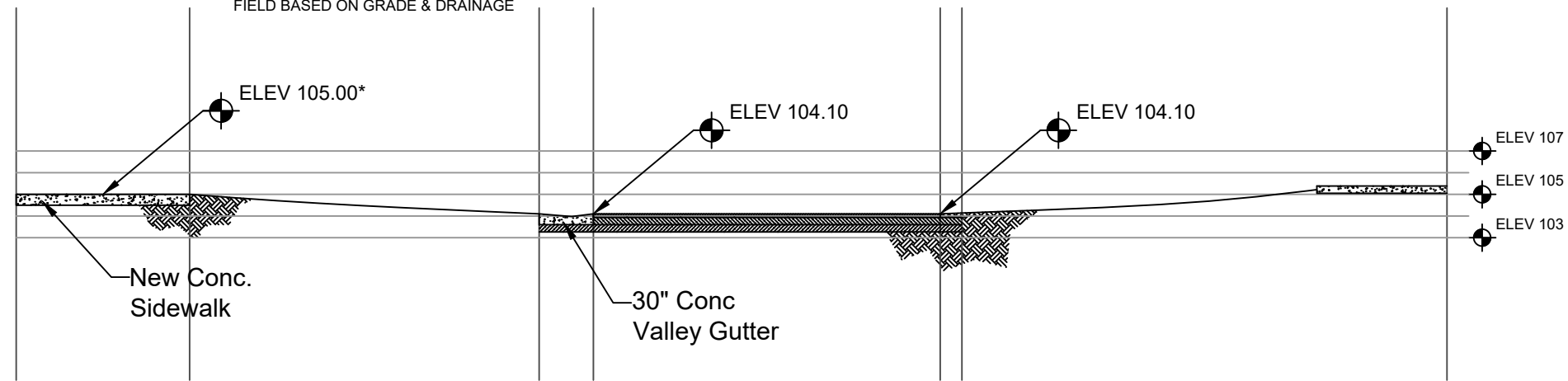
CROSS SECTION STA 02+00
