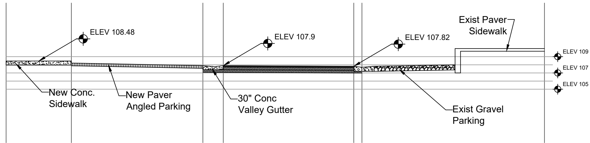
CROSS SECTION STA 00+50
