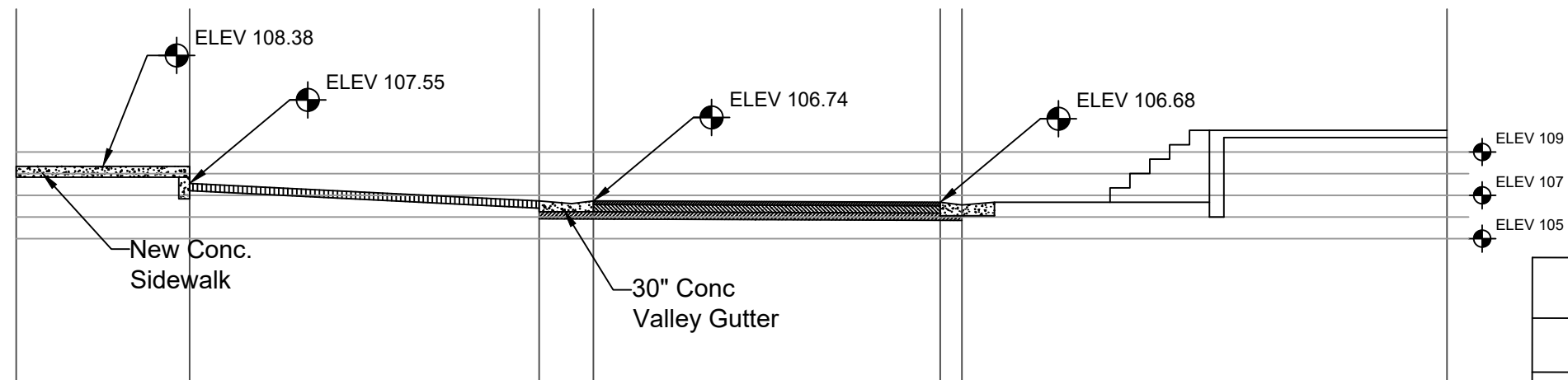
CROSS SECTION STA 01+00
