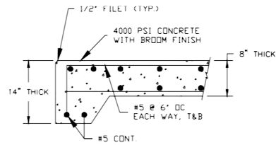
② GENERATOR SLAB DETAIL N.T.S.
