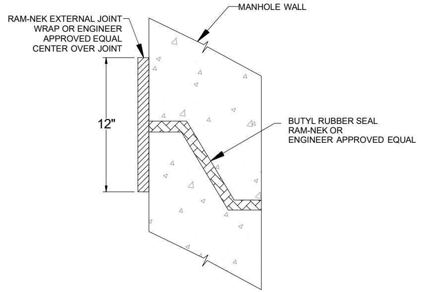
MANHOLE JOINT DETAIL N.T.S.
