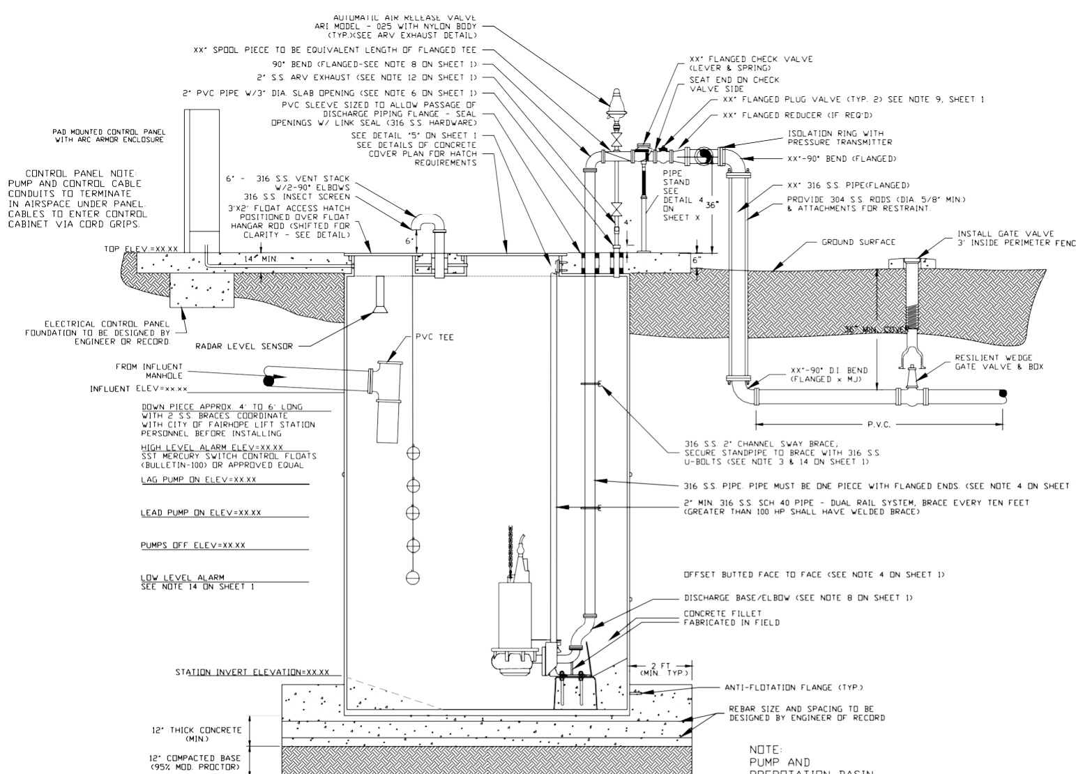
CROSS SECTION AA N.T.S.
