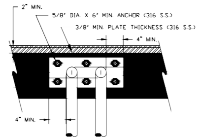
⑥ GUIDE RAIL N.T.S.
